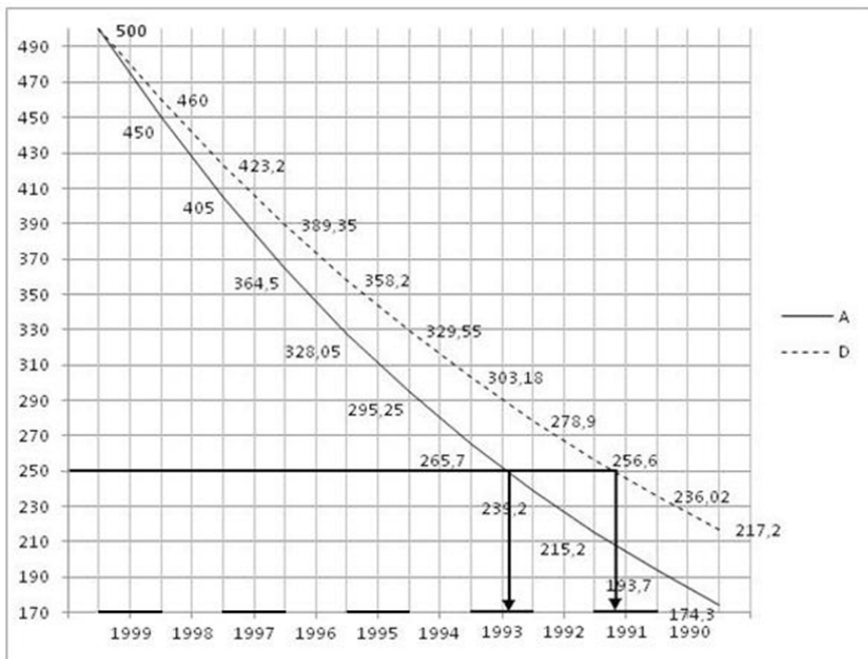
Wykres 3. Różnica pomiędzy okresem half-life skorygowanym i nieskorygowanym. Dane przykładowe opracowane na podst. Line, 1970
